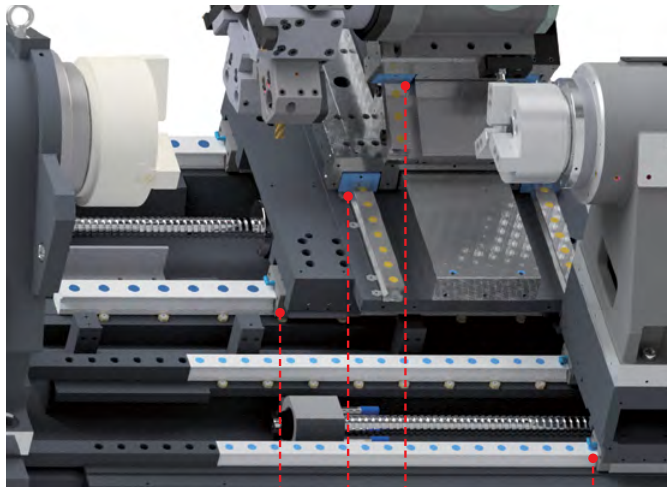
Roller Type LM Guide
