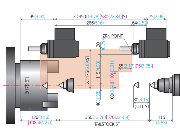
Angular milling head(ER25)
